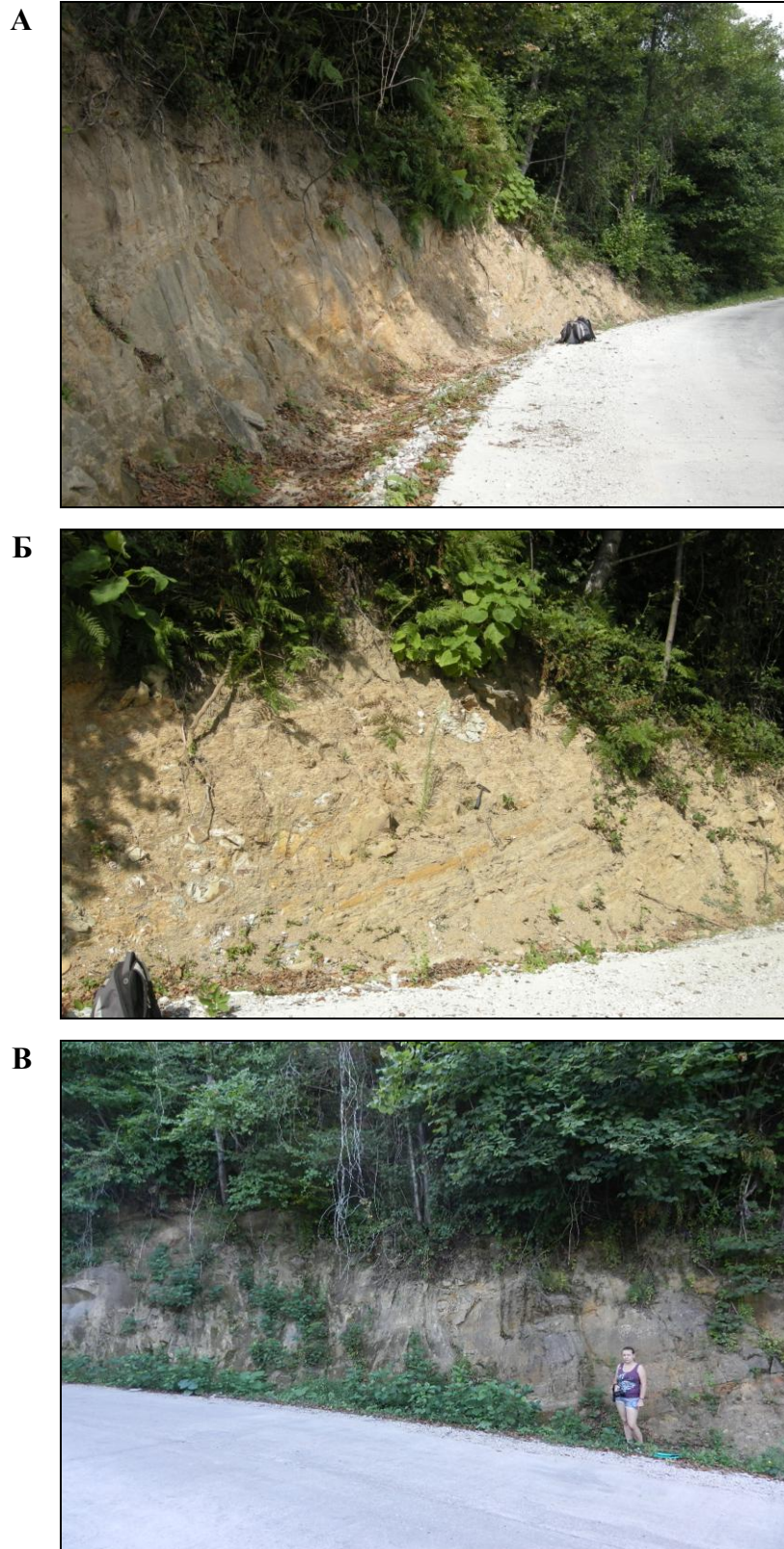
Рис. 4.25. Вид обнажения склонового канала-2 олигоцена (майкопская серия). А – общий вид обнажения. Выделяется три пачки. Пачка 1 – переслаивание маломощных турбидитовых песчаников и глин. Пачка 2 – толща дебритов с фрагментами неокатаных осадочных пород, толщина 1,5 м (Б). Пачка 3 – толща бесструктурных песчаников (В); в пачке имеются тонкие прослой глины и горизонтами с неокатанными кластами глины. Пачка образована амальгамацией нескольких слоев песчаников. Район г. Адлер, с. Шиловка.
