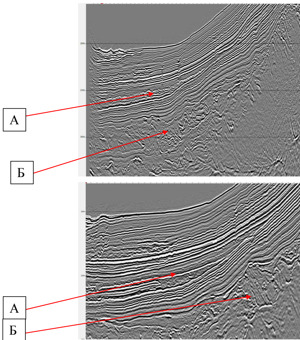
Рис. 3.16. Фрагмент сейсмического профиля для района в дельте Нигера. А – вероятная толщина отложений транспорта масс. Так как она выклинивается вверх по склону, то вероятно предположить ее образование в эпоху низкого стояния моря, для которой типично формирование обломочных потоков на склоне. Б – горизонт с крупными телами оползневого потока; наклонные рефлекторы могут быть взбросами в нижней части склона с нагромождением оползших тел.
