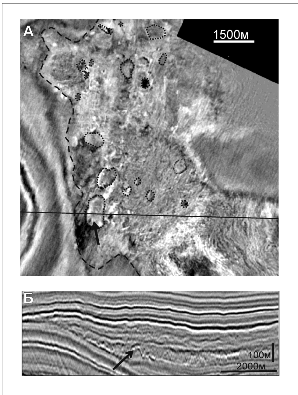
Рис. 3.20. Слайс по сейсмическому кубу для склона вала Шатского в Черном море (А) и сейсмический разрез к нему (Б). На рис. А пунктиром оконтурены отдельные вероятные олистолитовые тела. Стрелкой показано одно и то же тело на слайсе и разрезе. [Митюков и др., 2012].
