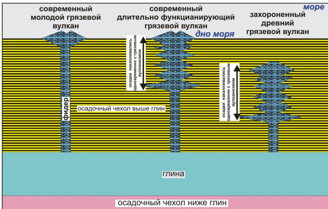
Рис. 6.6. Схемы строения грязевых вулканов [Никишин и др., 2011].
