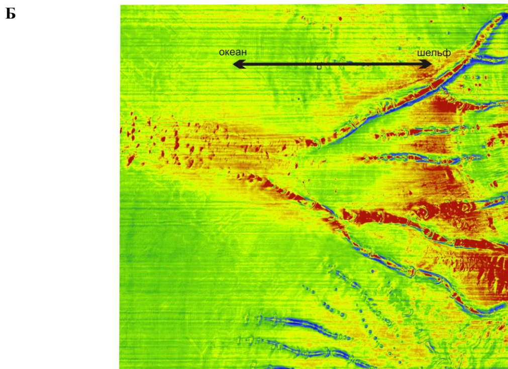
Рис. 4.8. Рельеф дна континентального склона участка в Экваториальной Африке (А) и карта RMS-амплитуд для интервала дно +50 мсек (Б). Каналы в целом прямолинейные, без меандр. Имеются отдельные кратероподобные формы – «покмарки» (rockmarks – «оспины»). Такие кратеры образуются прорывающимися газами или флюидами; иногда они выстраиваются в цепочки. На картах видно, что многие каналы начинаются на склоне.
