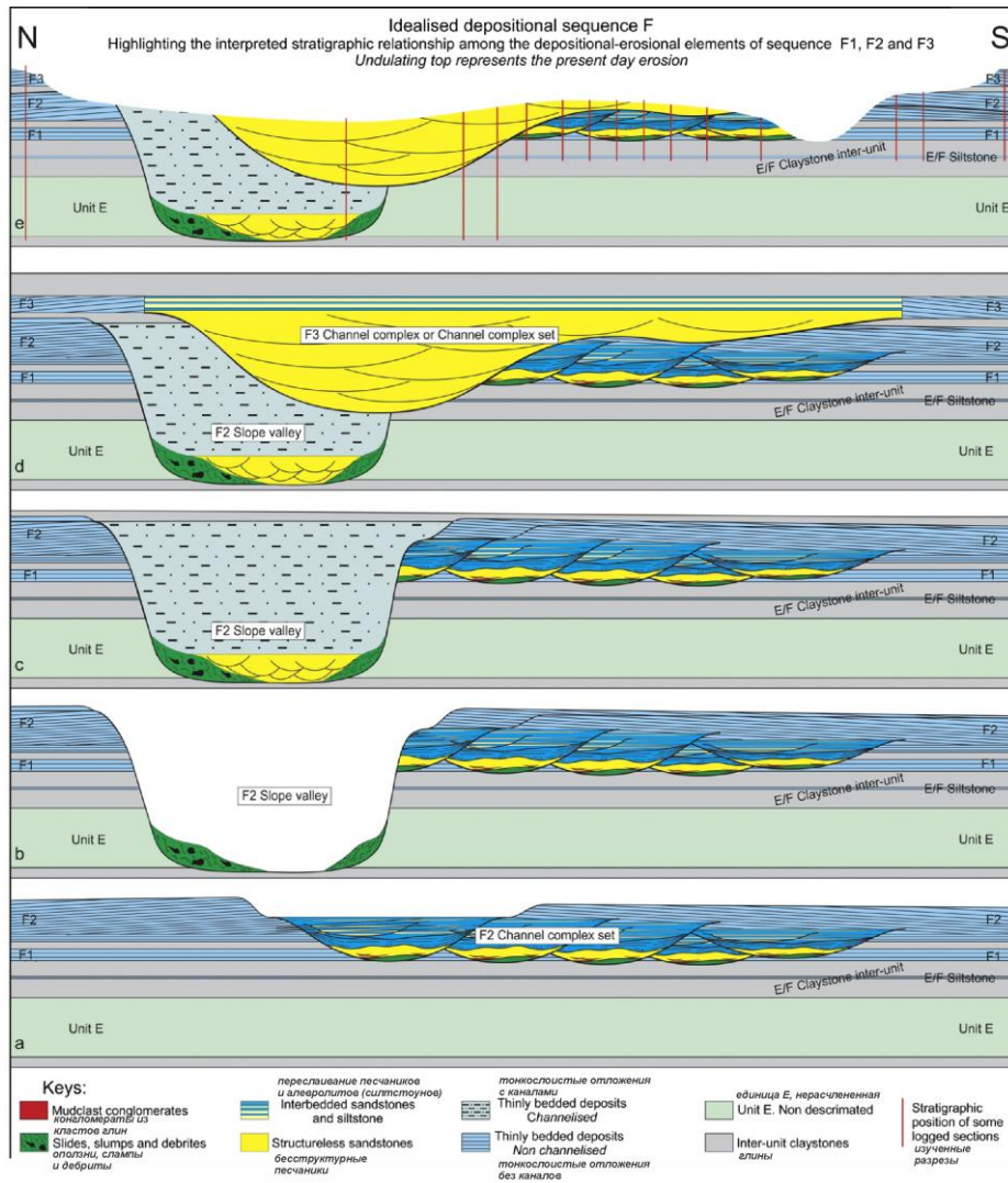
Рис. 5.10. Пример восстановления истории формирования глубоководной канальной системы, возникшей на палеосклоне в бассейне Кару в Южной Африке (формация Fort Brown, единица F). (a) Отложение секвенции F1 и начало стадии F2. Канальный комплекс сформировался в эту фазу. (b) Формирование склонового канала. (c) Формирование агградационной секвенции F2 с заполнением канала и последующее трансгрессивное перекрытие всей системы глинами в фазу высокого стояния уровня моря. (d) Формирование секвенции низкого уровня моря F3. (e). Современный разрез. Данный пример хорошо иллюстрирует возможный сценарий истории формирования канальных систем, хорошо видных по данным 3D сейсморазведки.
