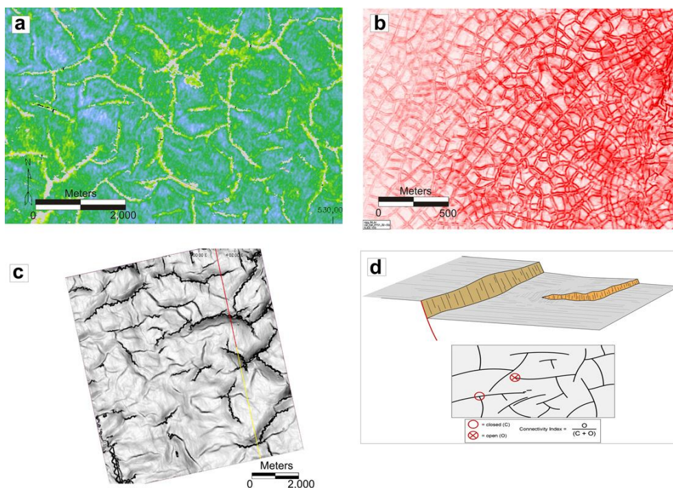
Рис. 6.3. Горизонтальные сейсмические слайсы для районов с полигональными системами разломов. В плане разломы образуют полигональный структурный рисунок. Рисунок (d) схематически показывает соотношение разных разломов. [Cartwright, 2011].
