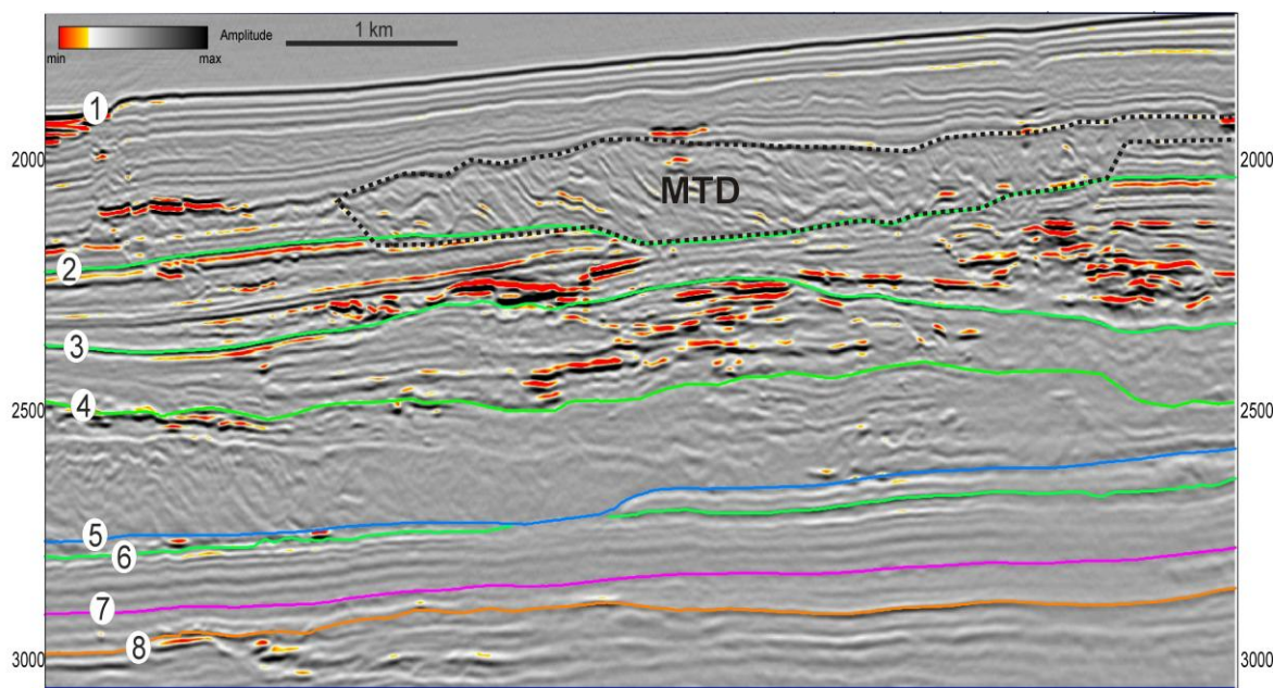
Рис. 3.19. Фрагмент сейсмического профиля для района континентальной окраины Африки. МТД – отложения транспорта масс. Отражения внутри МТД в нижней части палеосклона образуют системы надвигов, вероятно, в глинистой массе.
