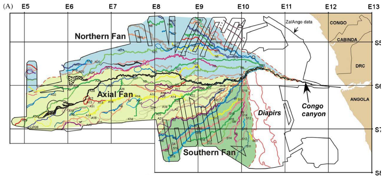
Рис. 4.2. Вверху показан рельеф дна Атлантического океана для глубоководного продолжения дельты реки Конго (Заир). Видно, что канално-фэновая система простирается более чем на 700 км от берега [Babonneau et al., 2002]. Внизу показана схема строения этого региона [Savoie et al., 2009].
