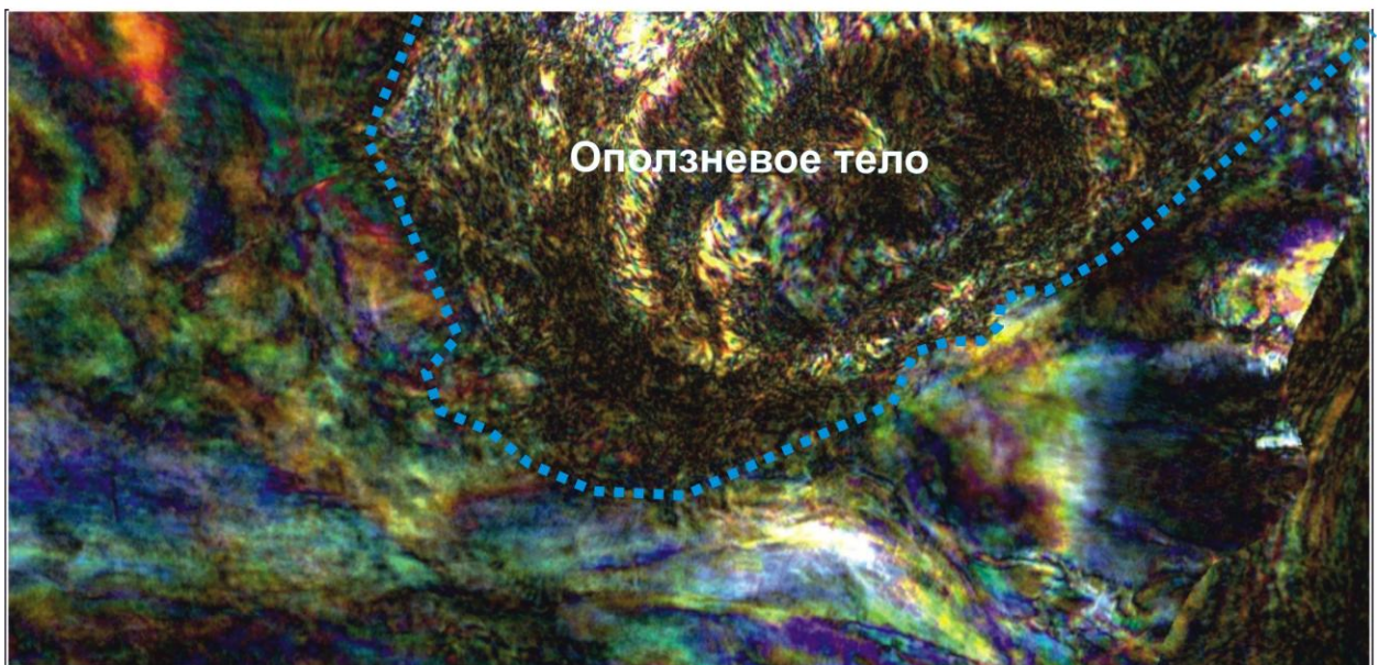
Рис. 3.25. Вид на разрезе и сейсмическом слайсе оползневого тела Понгве. Континентальная окраина Экваториальной Гвинеи.
