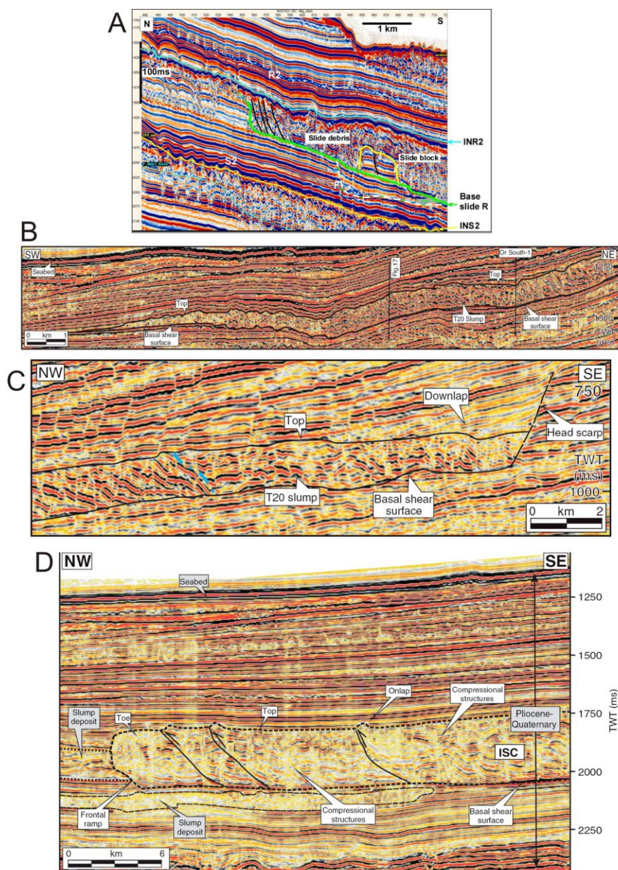
Рис. 3.15. Примеры интерпретации отложений транспорта масс на сейсмических профилях. А – фрагмент профиля для района оползневой потока Сторегга на континентальном склоне Норвегии. Это верхняя часть склона, для которого характерно оползание и сопутствующее растяжение. Видны сбросы, вероятные обломочные потоки (slide debris) и крупные оползшие блоки (slide block, или олистолит). [Solheim et al., 2005]. В, С, D – фрагменты профилей для континентального склона Средиземного моря в Израиле. [Frey-Martinez et al., 2006]. Хорошо видны оползневые потоки (slumps), на “D” четко видны взбросы и структуры сжатия в потоке.
