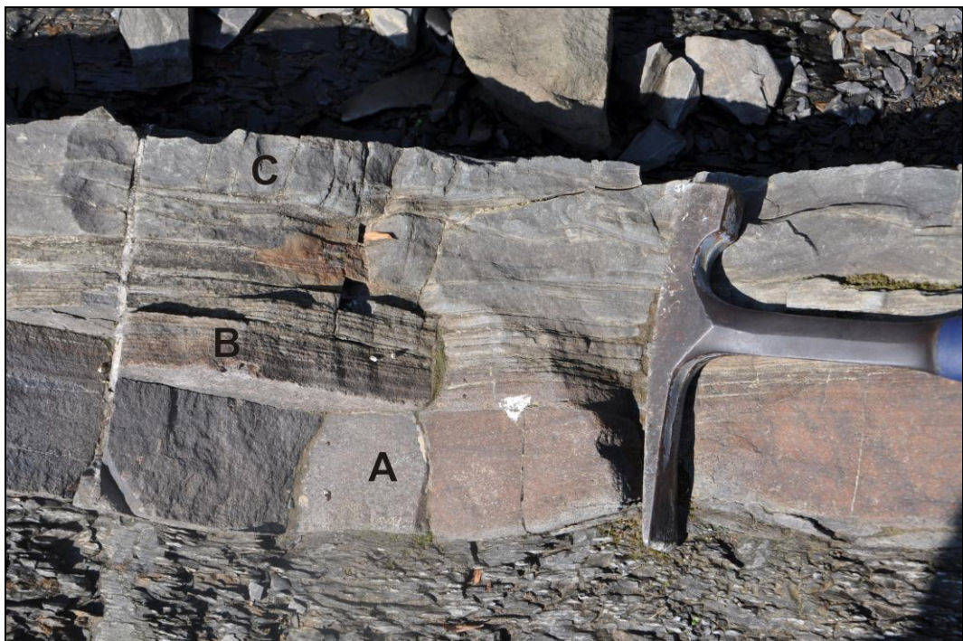
Рис. 2.3. Секвенция турбидитовых песчаников. А – бесструктурные песчаники, В – песчаники с параллельной слоистостью, С – песчаники с разнообразными текстурами. Породы таврической серии верхнего триаса - нижней юры в районе с. Прохладное, река Бодрак (Горный Крым).
