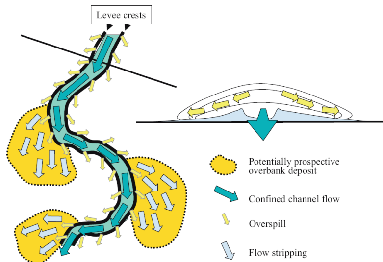
Рис. 4.46. Схема строения канала с «леви» (leveed channel) в плане и в разрезе. На разрезе видно, что турбидитовый поток располагается над гребнем «леви». В местах изгиба канала турбидитовый поток может продолжать прямолинейное движение и образовывать осадок на поверхности «леви» с повышенным количеством песка (overbank deposits – отложения поверх поднятия, наложенные отложения).
