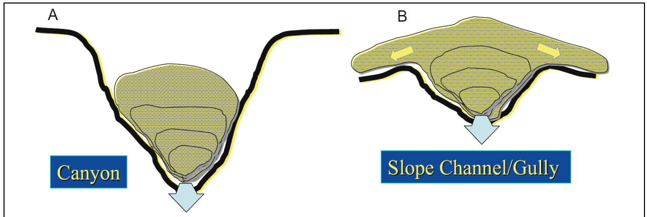
Рис. 4.4. Схематические разрезы через каньон (A) и склоновый канал (B). Осадочные процессы в каньоне целиком ограничены его стенами, осадки «леви» не образуются вокруг каньона. В каналах, наоборот, осадки не ограничены его стенами, и осадки типа «леви» наблюдаются вокруг канала. [Posamentier, Walker, 2006].
