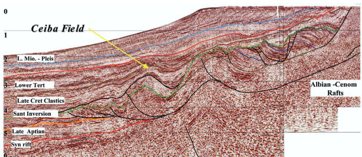
Рис. 6.16. Интерпретация сейсмического разреза для пассивной окраины Африки в Экваториальной Гвинеи. Отложения альба-верхнего мела оползли по толще солей, образуя на дне моря относительные поднятия. Одно из таких поднятий препятствовало транспорту турбидитового материала в позднем мелу, и перед ним накопилось относительно большое количество турбидитовых песчаников. Песчаники стали резервуаром для месторождения Сейба [Dailly et al., 2002].
