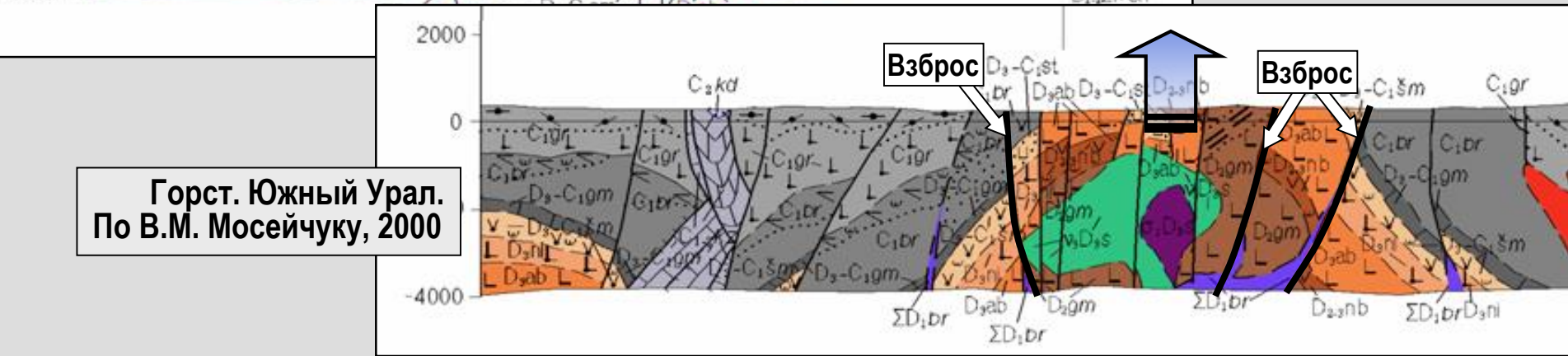
Рамп. Южный Урал. По В.М. Мосейчуку, 2000
