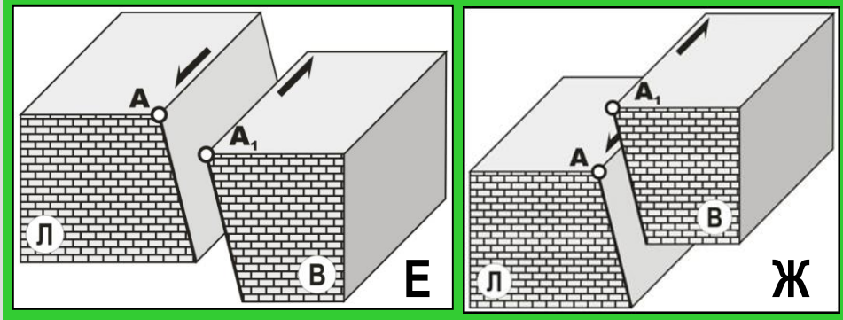
Комбинированные разрывы: Е – сбросо-сдвиг; Ж – взбросо-сдвиг.
